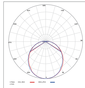
120 DEGREE(PC LENS)
